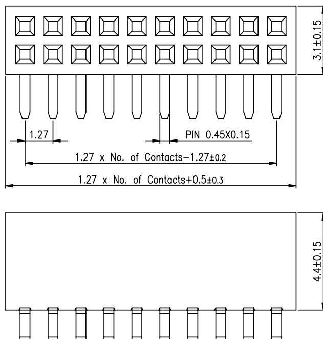
DIMENSIONS UNIT:mm EBB15-SDxxL
