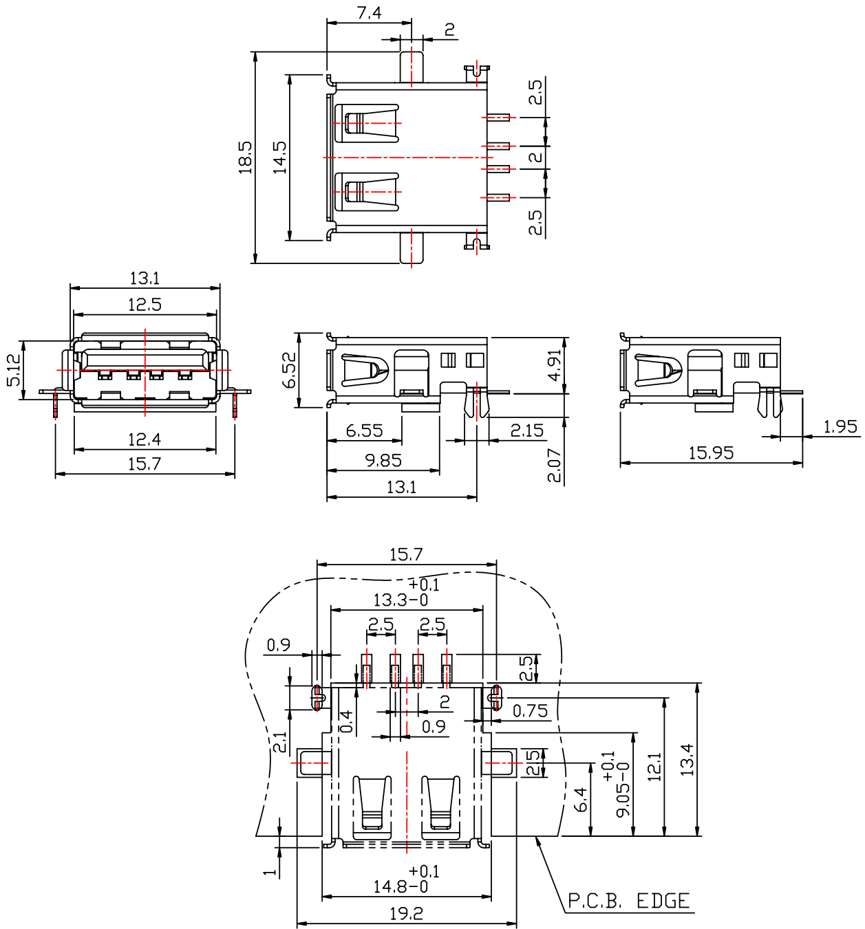
P.C.B. Layout
