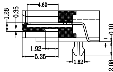
Sect A-A
