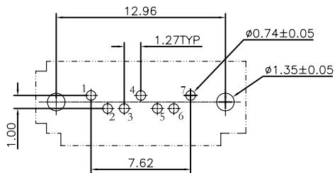
P.C.Board Layout
