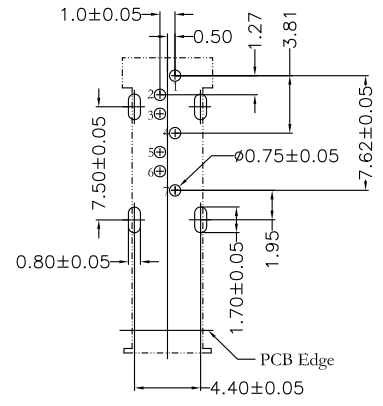
P.C.Board Layout
