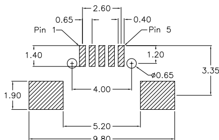
P.C.Board Layout
