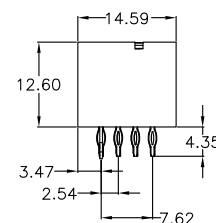
Press Fit Type
