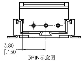
3PIN示意图
