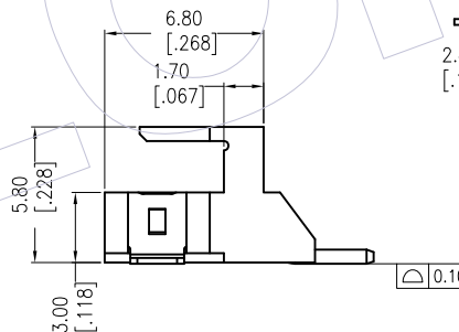
2PIN示意图
