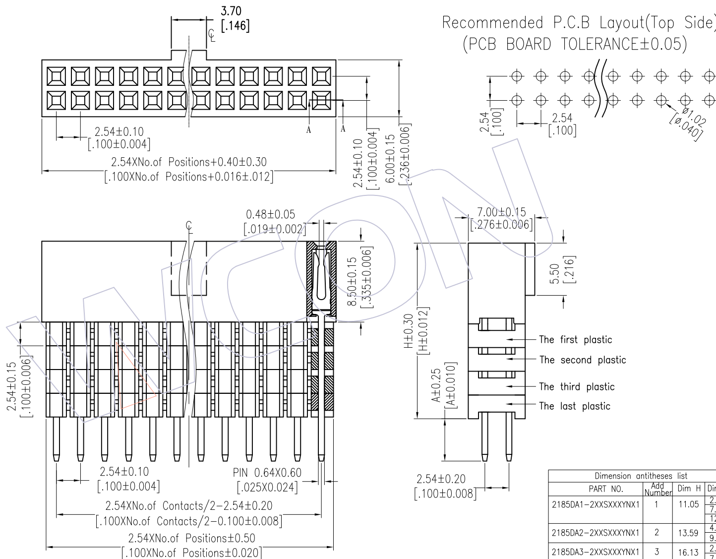
SECTION A-A
