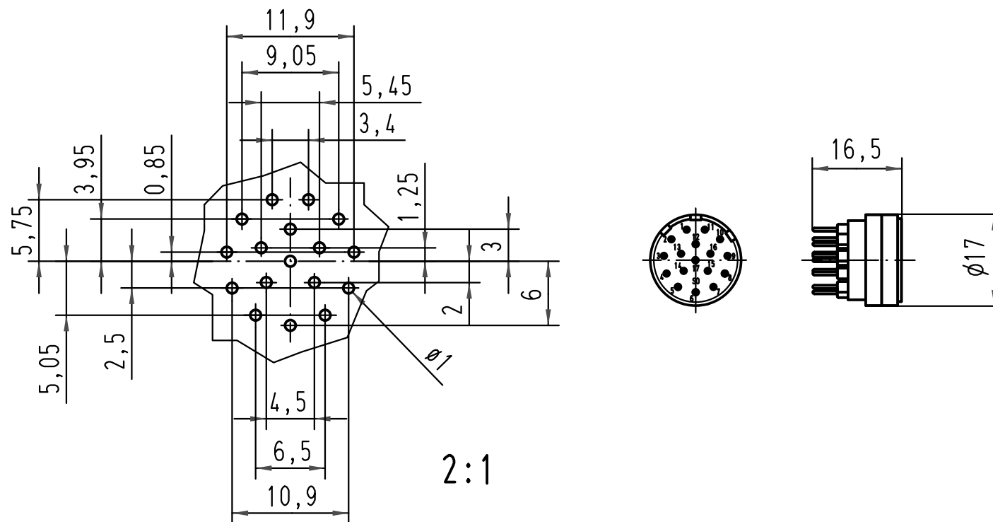
Lochbild/pinhole pattern
