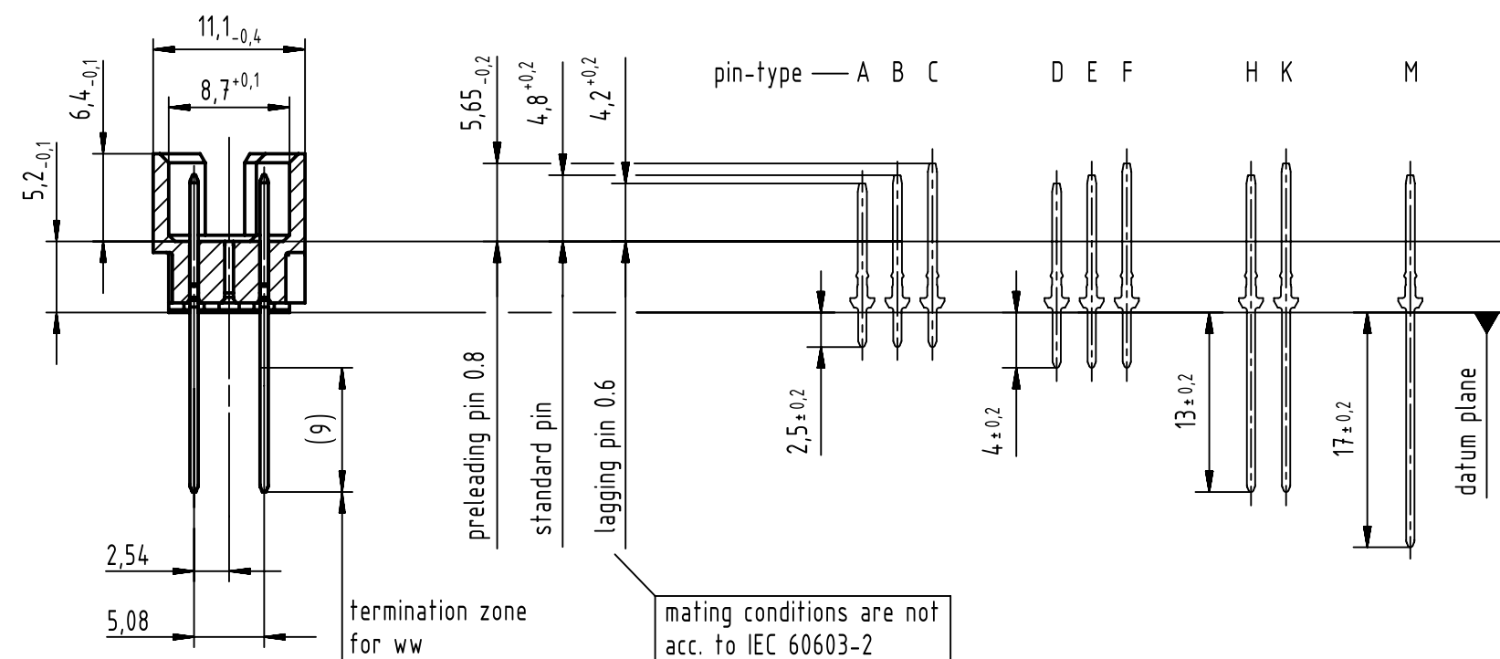
A-A (2:1)
