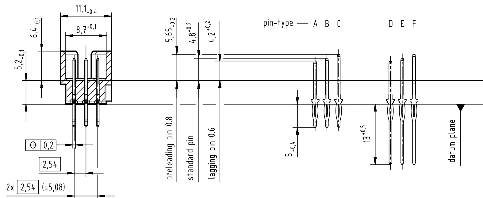
A-A (2:1)
