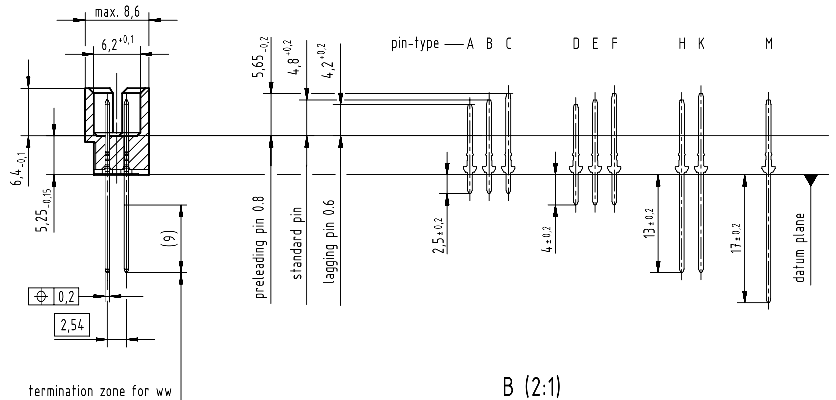
A-A (2:1)
