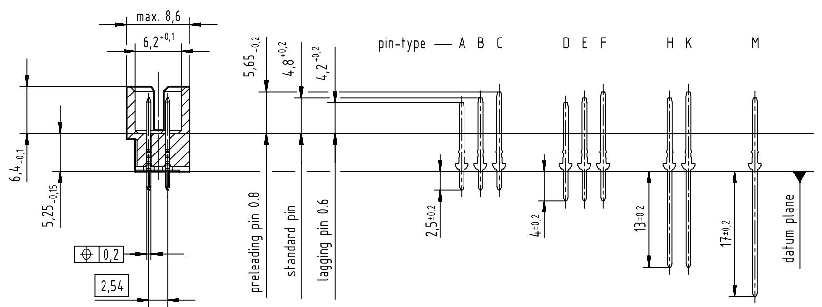
A-A (2:1)
