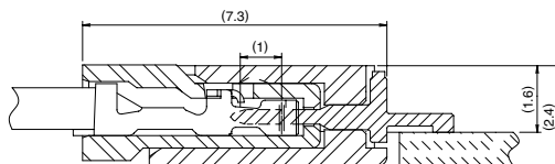
DF14H
